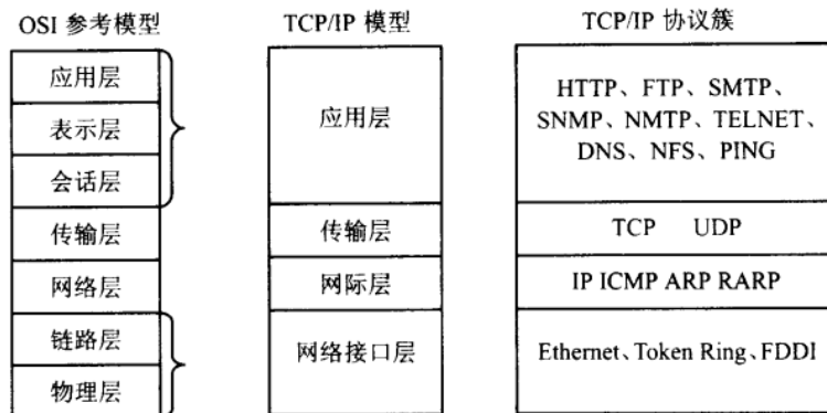
图 7-1 OSI 参考模型和 TCP/IP 协议对应关系
