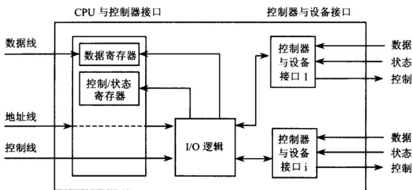
图 6-1 设备控制器的构成
