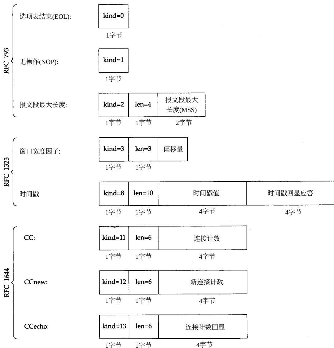
图2-1 TCP选项
